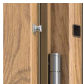
4 bezpečnostní trny proti vylovení
