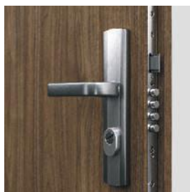
líštový vícebodový zámek přizpůsobený pro dvě cylindrické vložky
