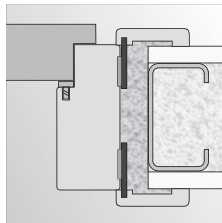
montáž na pěnu do stěny ze sádkokartonu
