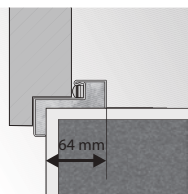
rohová zárubeň malá PLUS
