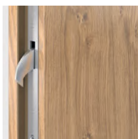
Háček – horní / dolní závora SAFE typ III, ENERGY PROTECT
