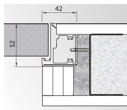
Bezpolodrážkové standard (otevírané ven)
