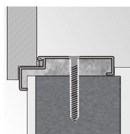
rohová zárubeň veľká montáž pomocou šroubov
