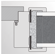
montáž na pěnu do zděné stěny
