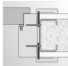
montáž na vruty do stěny ze sádkokartonu
