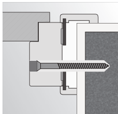
montáž na pěnu a kotvy do zděné stěny
