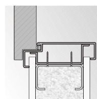
rohová zárubeň veľká montáž na sádkartónovú stenu
