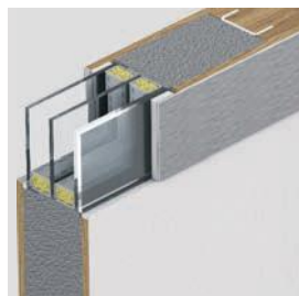
Dvoukomorové bezpečnostní prosklení třídy P4 a rám z nerezové oceli
